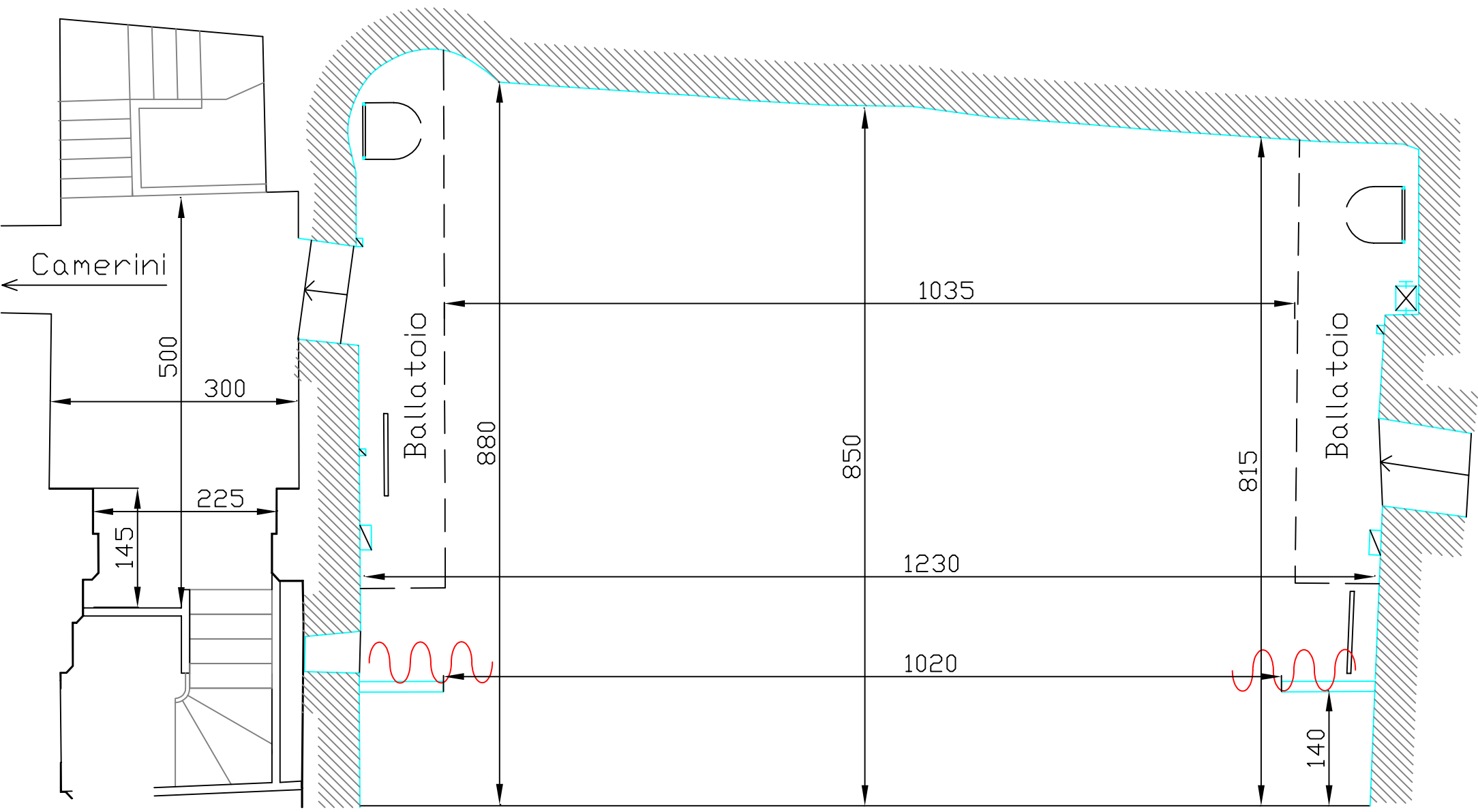
Planimetria palcoscenico Sala Umberto Roma - Declivio 2,75%
